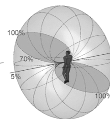
La radiación de una antena convencional 2,4 GHz
